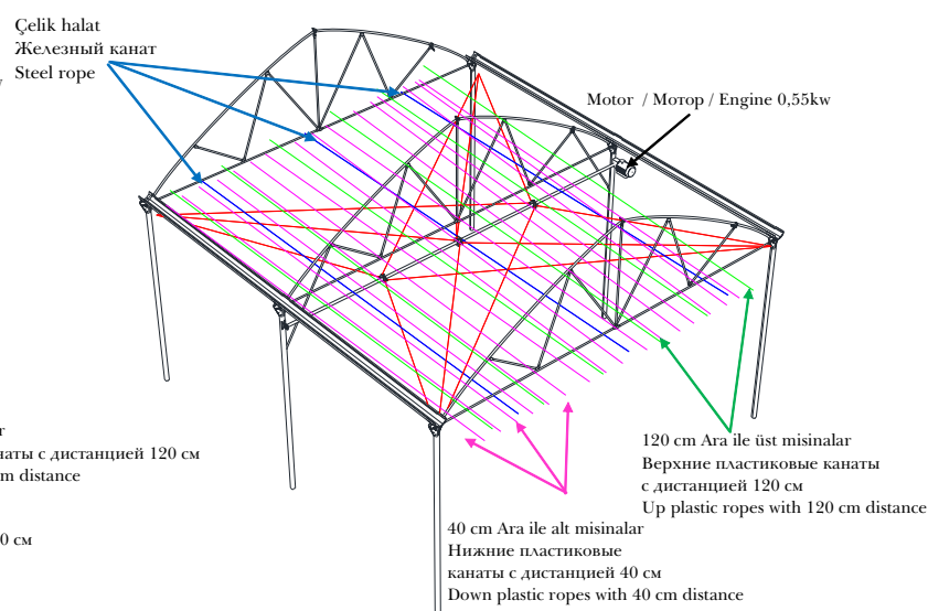
HALATLI PERDE SİSTEMİ STAINLESS SHADING SYSTEM ТРОСНАЯ СИСТЕМА ЗАШТОРИВАНИЯ
